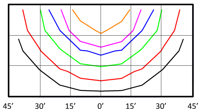
FLEDWPCA80W-5K (9,241 Lumens)
