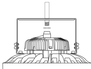
1/2" Conduit-Mounted (VICOHBRN-YOKE-PRM)
