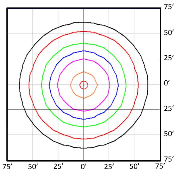
VICOHBR14-4K-B-UNV (13,961 Lumens)
