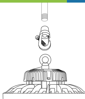
3/4" Conduit-Mounted VICOHBRN-PSH-PRM-V2)
